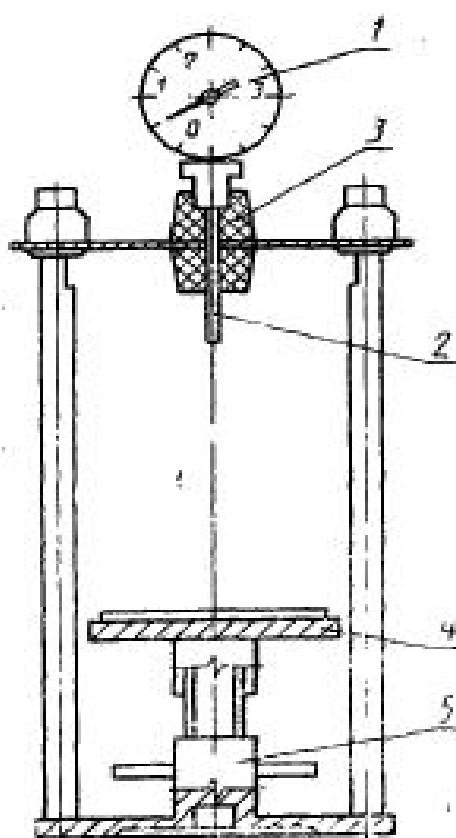
1 — манометр; 2 — игла; 3 — уплотнительная прокладка; 4 — площадка пресса; 5 — винт
